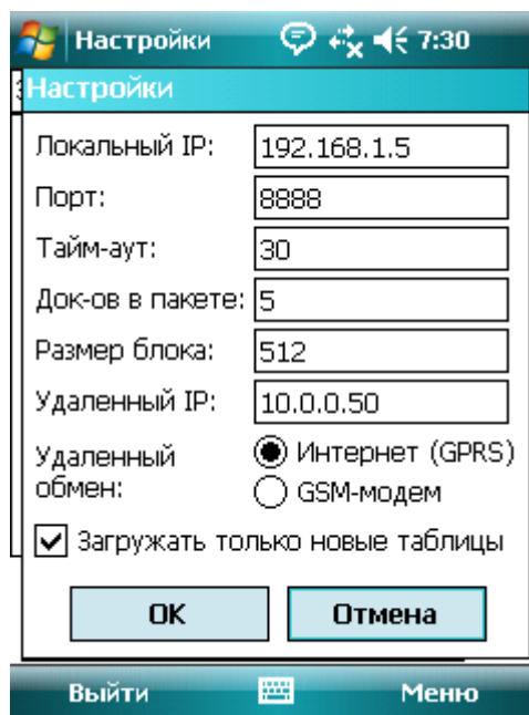
рис. 7.8 «Настройка приложения PalmClient»
